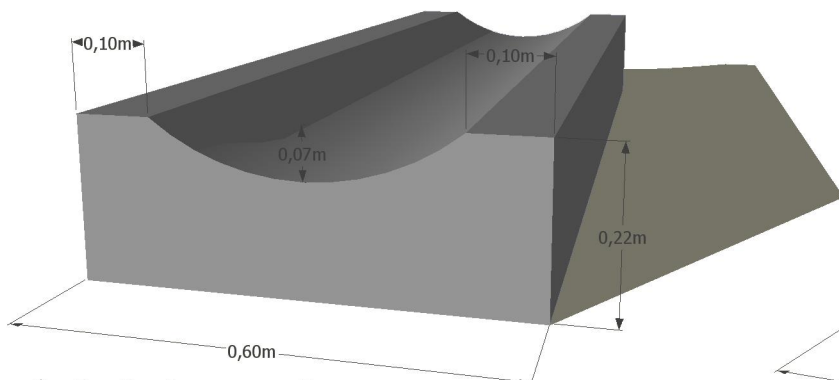
ściek korytkowy
